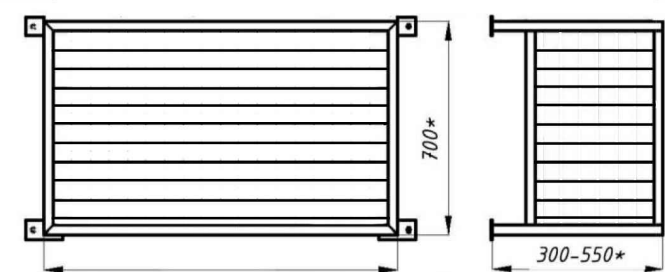
Чертеж декоративной решетки наружного блока
